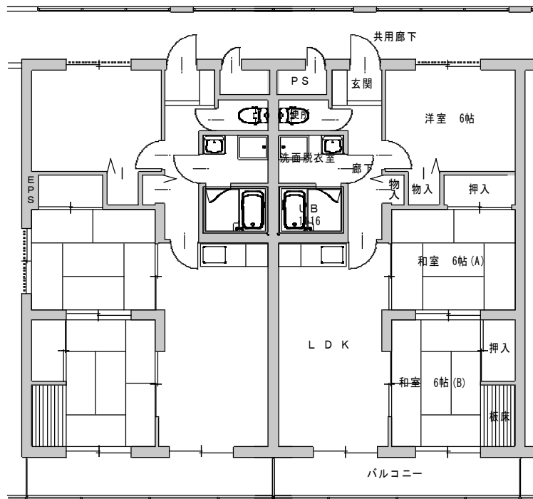
平面図
