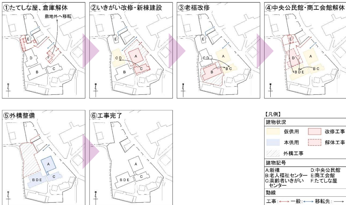
工事ローテーション【増改築】
