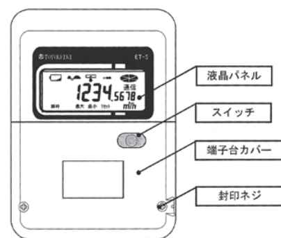
【端子台】
