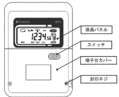
【端子台】
